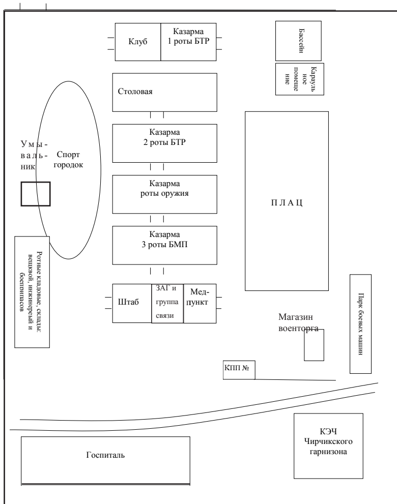
Общий план военного городка отряда в г. Чирчике.
